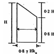
2. (Terzaghi-peck, 1948)
