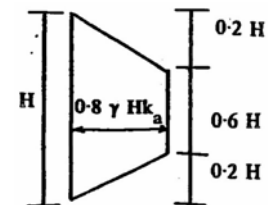
1. (Terzaghi-peck, 1948)
